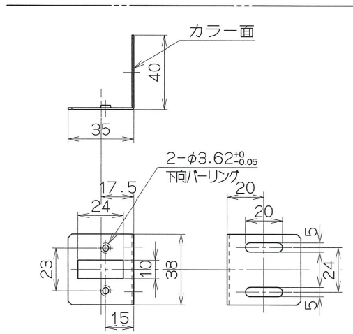
取付ベース
