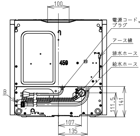
背面図
