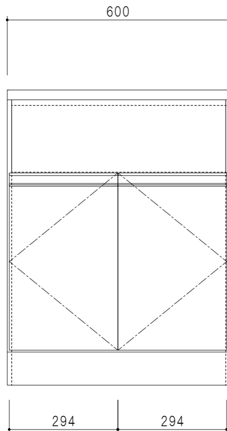
立面図
