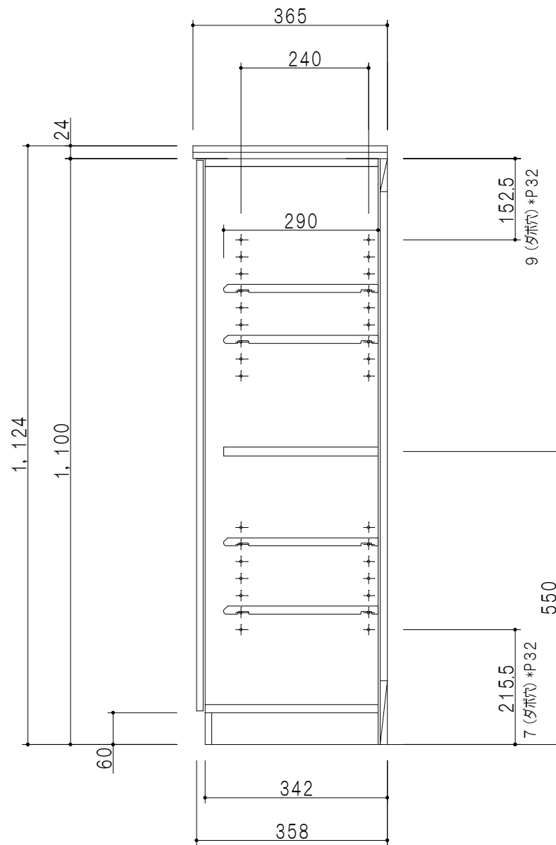
断面図
