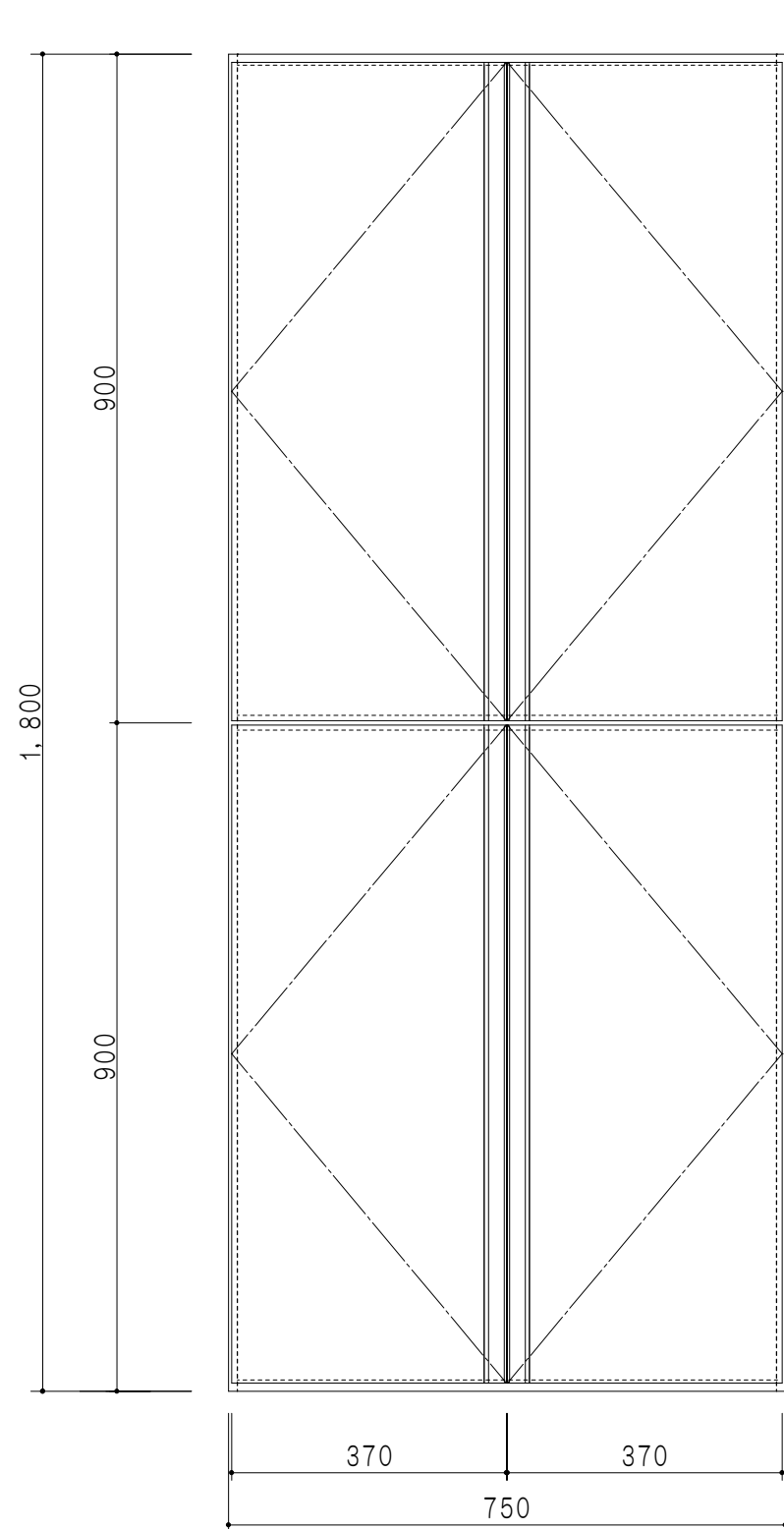
立面図
