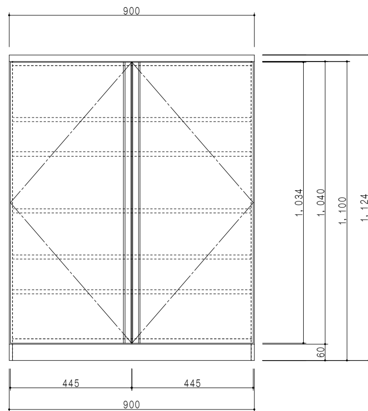
立面図
