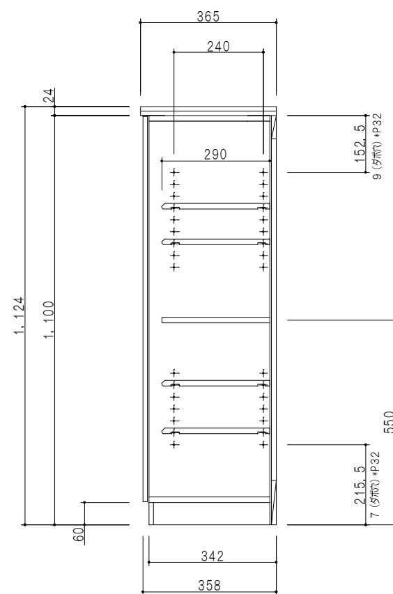
断面図
