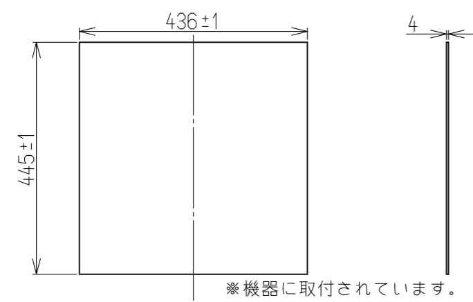
< ドア用化粧パネル寸法 > (上)
