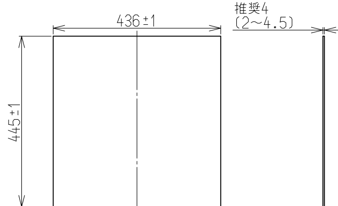
<ドア用化粧パネル寸法>(上)
